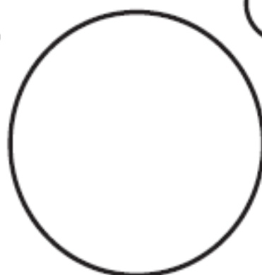
Uranus
