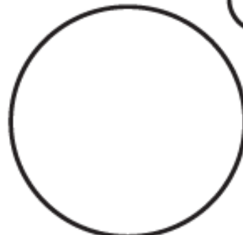
Venus
