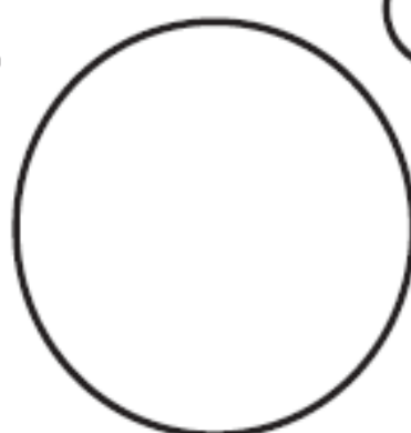
Jupiter
